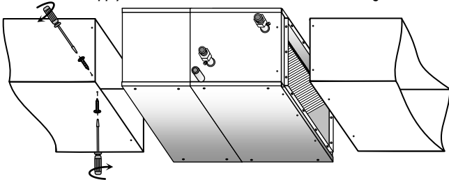
Bocca di aspirazione e mandata versioni "a vista": attacchi canale a baionetta Air intake and supply outlets of versions "with cabinet": duct nesting connections
